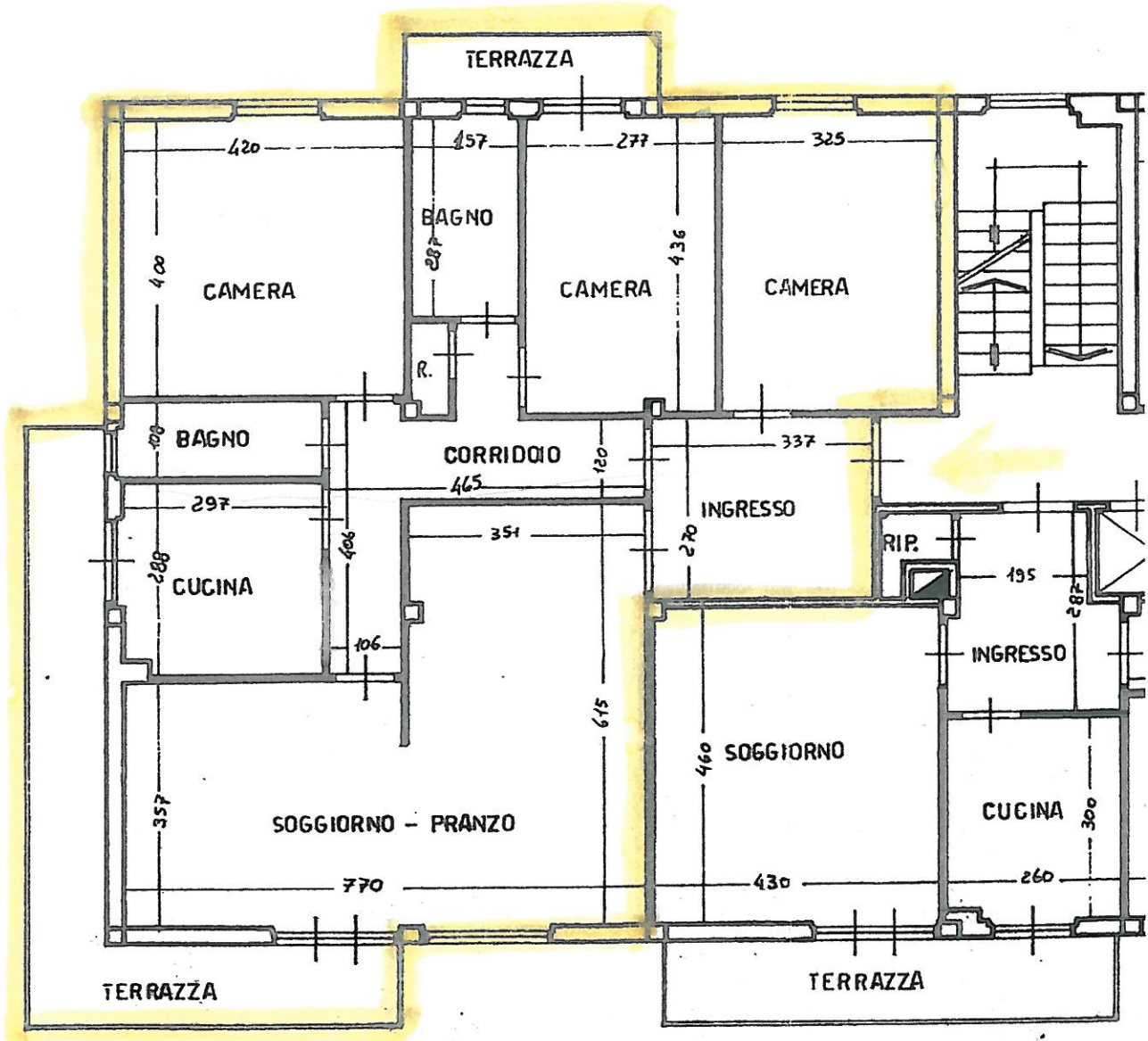
PIANO SECONDO H=3.00
