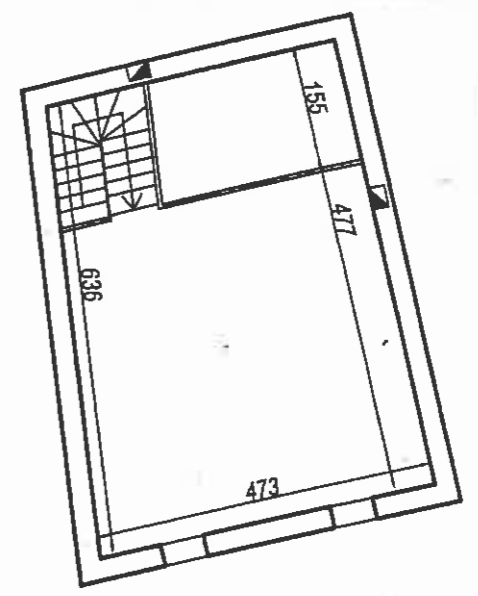
Pianta sottotetto
